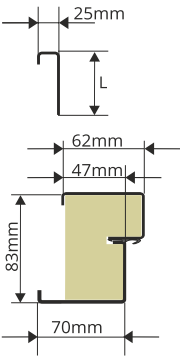
coup de profil Thermo ODS68
