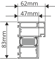
coup de profil Thermo ALU68
